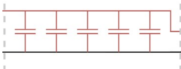
FIGURE 1.7 – Zoom sur le circuit de condensateurs
