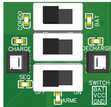
FIGURE 1.10 – Zoom sur l'interface de la carte principale du système d'allumage
