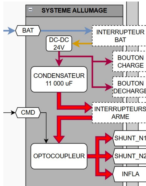
FIGURE 1.4 – Zoom sur le synopsis de la ligne de mise à feu (ref. annexe ??)
